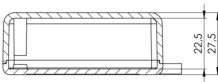
PRZEKRÓJ A-A
