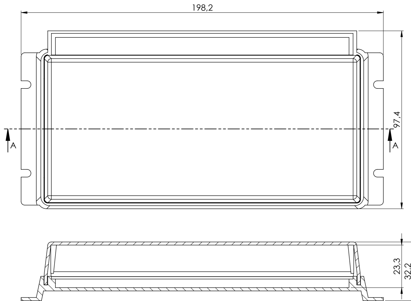
PRZEKRÓJ A-A
