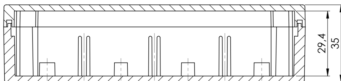
PRZEKRÓJ A-A
