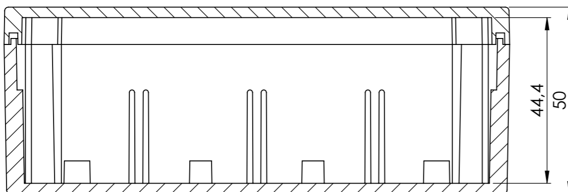
PRZEKRÓJ A-A
