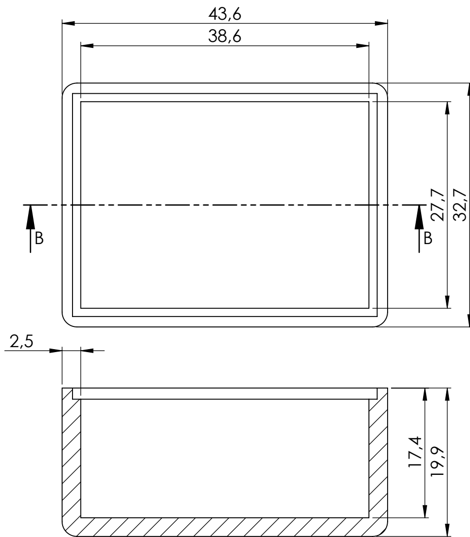
PRZEKRÓJ B-B
